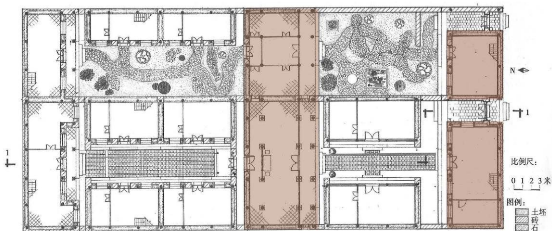
图 3-26 二号、三号民居的平面图及现存房屋
