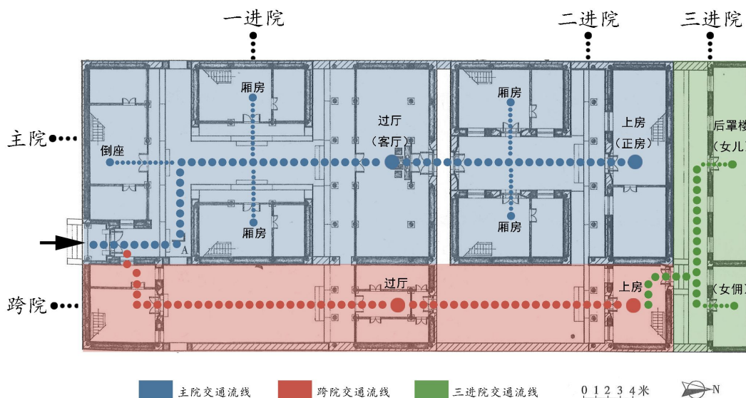
图 3-14 四号民居的平面布局及交通流线图
