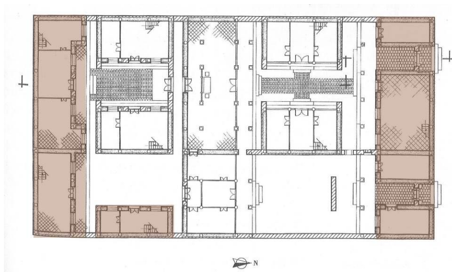
图 3-40 九号、十号民居的平面图及现存房屋
