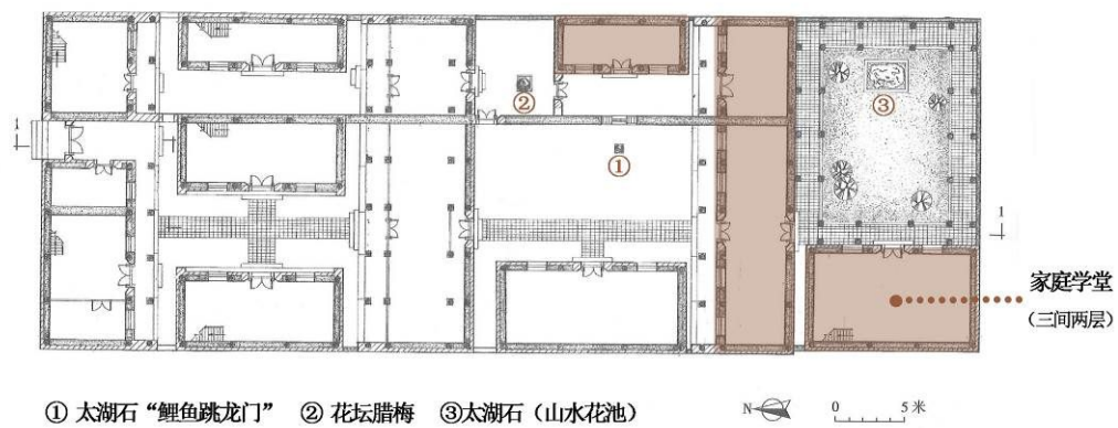
图 3-43 十五号民居的平面图及现存房屋
