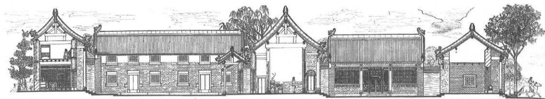
图 3-27 二号、三号民居的立面图（图片来源：左满常《河南民居》）
