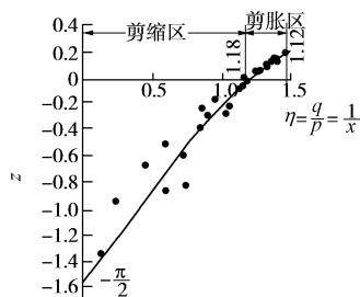
图 2 屈服函数中试验常数 r 与 k 的确定
