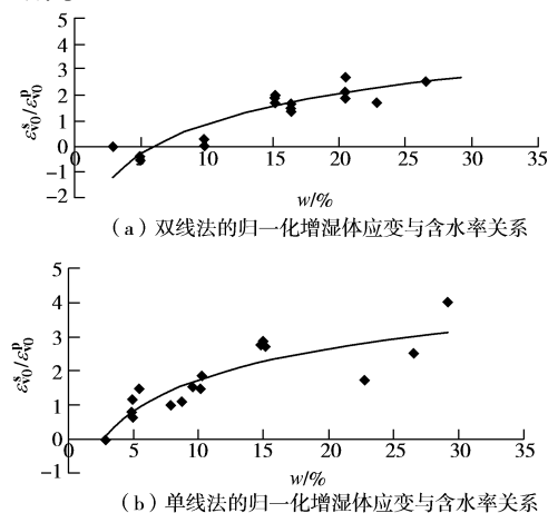
图 7 归一化增湿体应变 e_{v0}^s/e_{v0}^p 与含水率 w 关系曲线
