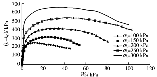
图 10 各种围压下试验得到的塑性功与硬化参数关系
