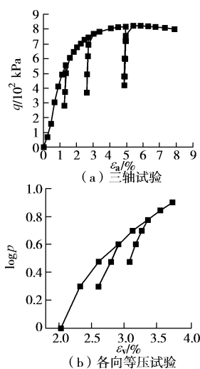
图 12 加载减载一半的循环加载试验结果
