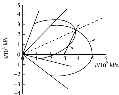
图 13 减载过程中的旋转硬化
