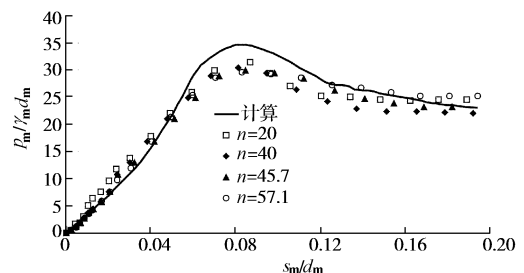
图 11 浅基础的渗水力模型试验的荷载沉降曲线与模型的有限元计算结果比较
