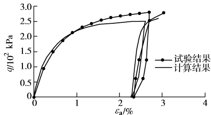
图 14 旋转硬化清华模型计算结果与试验结果对比
