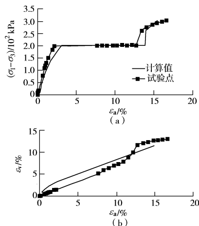
图 8 试验与计算的增湿试验结果
