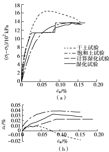
图 5 试验与计算的结果比较
