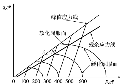
图 9 密实永定河砂的试验确定的屈服面
