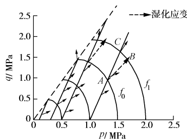
图 6 堆石料的屈服面与湿化应变的正交性
