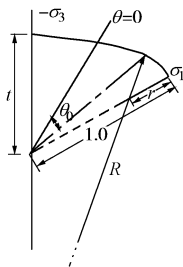
图 4 \pi 平面上的双圆弧屈服轨迹
