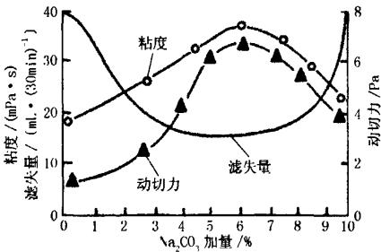
图 1 \text{Na}_2\text{CO}_3 加量对泥浆性能的影响
