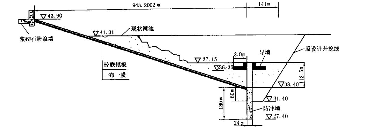
图1 土壤固化剂混凝土防冲墙标准断面图
