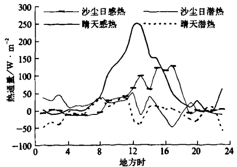
图 7 2006 年 8 月 31 日(晴天)与 17 日(沙尘日)塔中站感热、潜热对比曲线
