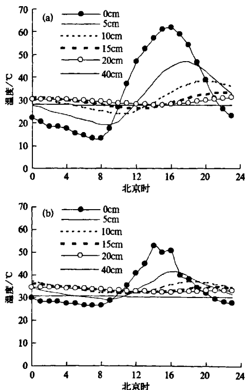
图5 2006年8月31日(晴天)与17日(沙尘日)塔中站地温日变化曲线 a. 晴天地温日变化; b. 沙尘日地温日变化
