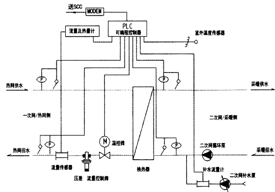
图2 供热站调控原理示意图
