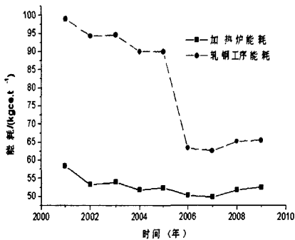
图 1 首钢近年轧钢系统工序能耗和加热炉能耗
