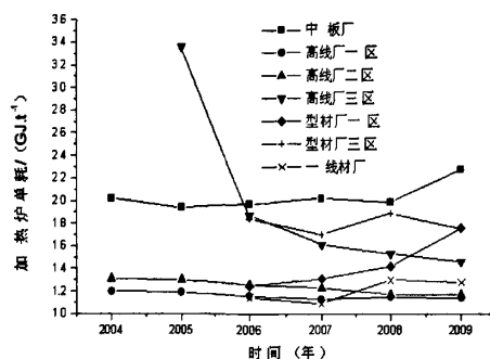
图2 首钢近年加热炉单耗变化
