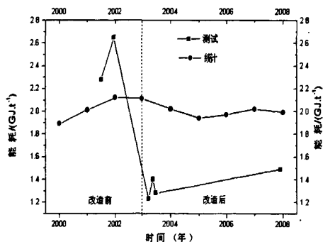
图3 中板厂2号加热炉热平衡测试与统计能耗对比
