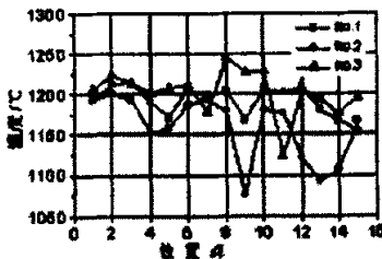
图 7 原加热炉钢坯表面温度分布
