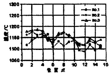
图 8 新加热炉钢坯表面温度分布
