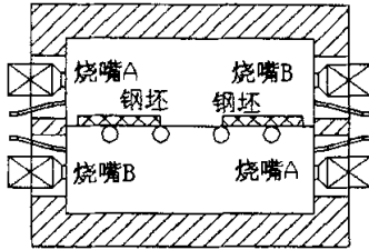
图 3 加热炉整体图
