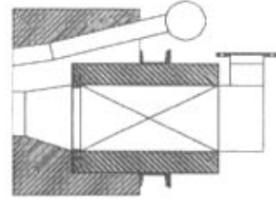
图 4 烧嘴方案
