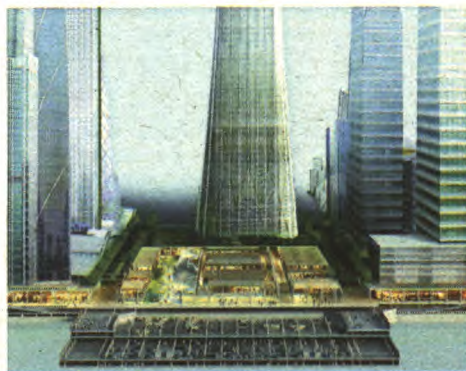
CBD核心区地下空间共五层,分别包括了地下交通系统、地下商业街、地下公共建筑、地下基础设施、地下储存空间、地下防御空间等。这是CBD核心区地下空间效果图。
